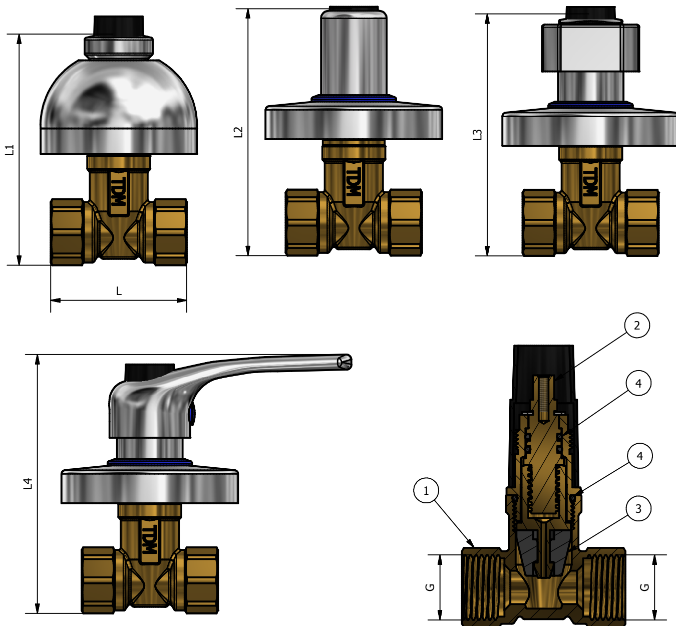
A-A ( 1 : 1.25 )
